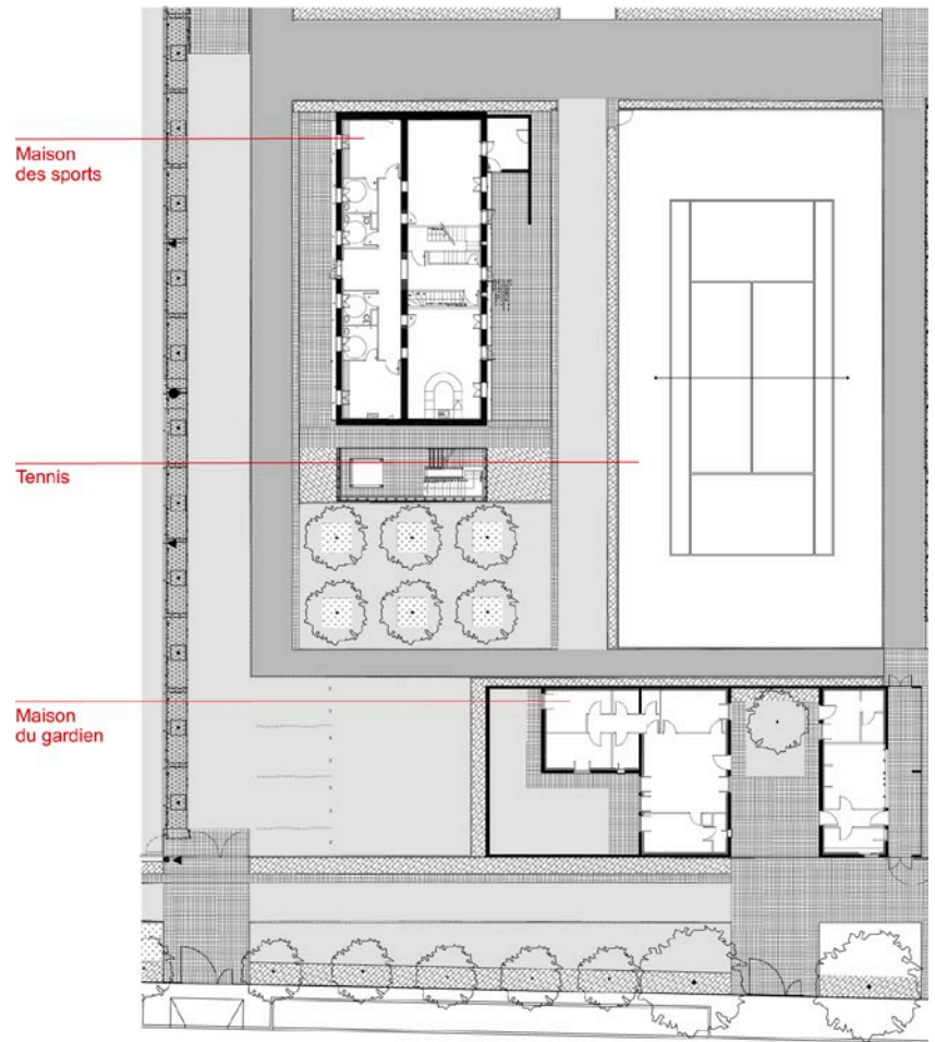
Plan Maison des Sports + Maison du Gardien
